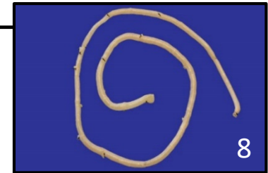
Allografts
